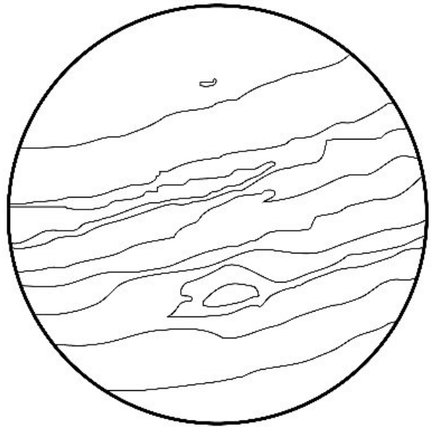
Jupiter
